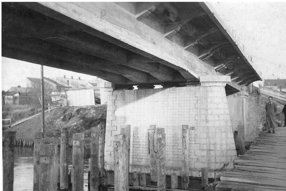
Lugoj - Construirea podului de beton (vedere de jos). Colecția Ing. Anton Tomin
