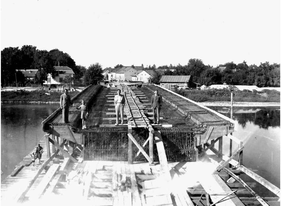
Lugoj - Construirea podului de beton (vedere parțială). Colecția Ing. Anton Tomin
